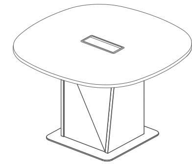
1000 (Dia) 1150 (Dia)
