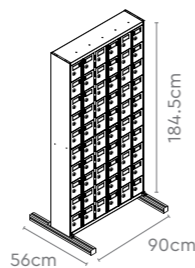
60 Door Locker Stand Fixed
